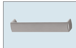
Nr. 673 Metallbügelgriff Edelstahl-Optik Bohrabstand 160 mm Überstand nach vorn: 29 mm
