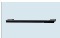
Nr. 753 Metallbügelgriff Schwarz Bohrabstand 160 mm Überstand nach vorn: 27 mm
