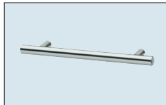
Nr. 629 Metallbügelgriff Edelstahl-Optik Bohrabstand 128 mm Überstand nach vorn: 33 mm
