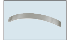
Nr. 744 Metallbügelgriff Edelstahl-Optik Bohrabstand 128 mm Überstand nach vorn: 30 mm
