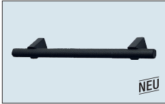
Nr. 764 ★ Metallbügelgriff Schwarz Bohrabstand 128 mm Überstand nach vorn: 29 mm
