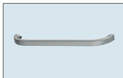
Nr. 712 Metallbügelgriff Edelstahl-Optik Bohrabstand 160 mm Überstand nach vorn: 30 mm
