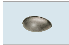
Nr. 751 Metallmuschelgriff Verzinkt Antik Bohrabstand 64 mm Überstand nach vorn: 25 mm
