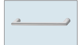
Nr. 706 Metallbügelgriff Edelstahl- Optik Bohrabstand 160 mm Überstand nach vorn: 32 mm
