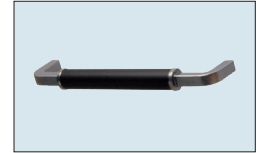
Nr. 774 * Bügelgriff Anthrazit gebürstet/ Schwarz Bohrabstand 160 mm Überstand nach vorn: 36 mm
