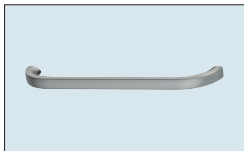
Nr. 712 Metallbügelgriff Edelstahl- Optik Bohrabstand 160 mm Überstand nach vorn: 30 mm
