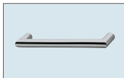
Nr. 705 Metalen beugelgreep rvs- decor Boorafstand: 160 mm Overstek naar voren: 41 mm
