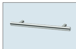
Nr. 629 Metalen beugelgreep rvs- decor Boorafstand: 128 mm Overstek naar voren: 33 mm
