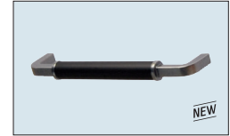
Nr. 774 * Beugelgreep antraciet geborsteld/zwart Boorafstand: 160 mm Overstek naar voren: 36 mm
