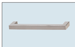
Nr. 702 Metalen beugelgreep rvs- decor Boorafstand: 128 mm Overstek naar voren: 41 mm
