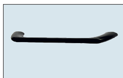
Nr. 762 Metalen beugelgreep zwart Boorafstand: 160 mm Overstek naar voren: 28 mm
