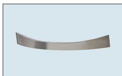
Nr. 695 Metalen beugelgreep rvs- decor Boorafstand: 128 mm Overstek naar voren: 30 mm
