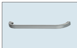
Nr. 712 Metalen beugelgreep rvs- decor Boorafstand: 160 mm Overstek naar voren: 30 mm
