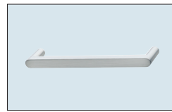
N° 690 Poignée arc métallique aspect inox Entraxe perforations : 128 mm Saillie vers l'avant : 35 mm
