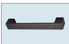
N° 757 Poignée arc métallique aspect fer antique Entraxe perforations : 160 mm Saillie vers l'avant : 28 mm
