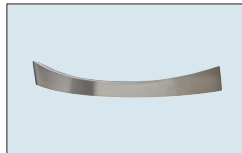
N° 695 Poignée arc métallique aspect inox Entraxe perforations : 128 mm Saillie vers l'avant : 30 mm
