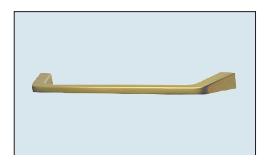
N° 772 Poignée arc métallique aspect doré Entraxe perforations : 160 mm Saillie vers l'avant : 27 mm
