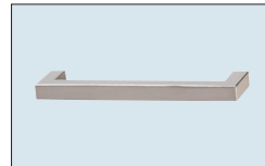
N° 702 Poignée arc métallique aspect inox Entraxe perforations : 128 mm Saillie vers l'avant : 41 mm
