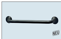
N° 781 Poignée arc métallique noir Entraxe perforations : 160 mm Saillie vers l'avant : 30 mm
