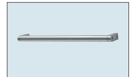
N° 723 Poignée arc métallique aspect inox Entraxe perforations : 160 mm Saillie vers l'avant : 35 mm
