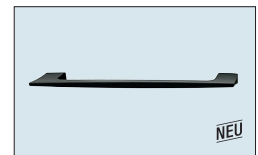
N° 782 Poignée arc métallique noir Entraxe perforations : 160 mm Saillie vers l'avant : 30 mm
