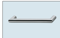
N° 705 Poignée arc métallique aspect inox Entraxe perforations : 160 mm Saillie vers l'avant : 41 mm
