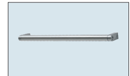
Nr. 723 Metalen beugelgreep rvs-decor Boorafstand: 160 mm Overstek naar voren: 35 mm
