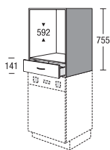
Opzetkast voor oven
