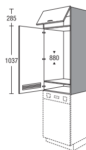
Opzetkast voor inbouwapparaat
