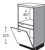
Highboard voor inbouwapparaten
