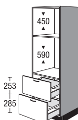
Hoge kast voor inbouwapparaten
