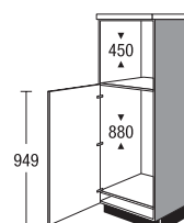
Highboard voor inbouwapparaten
