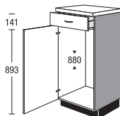
Highboard voor inbouwapparaten
