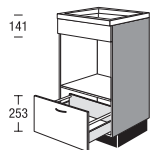
Onderkast voor inbouwapparaten
