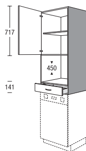
Opzetkast voor magnetron
